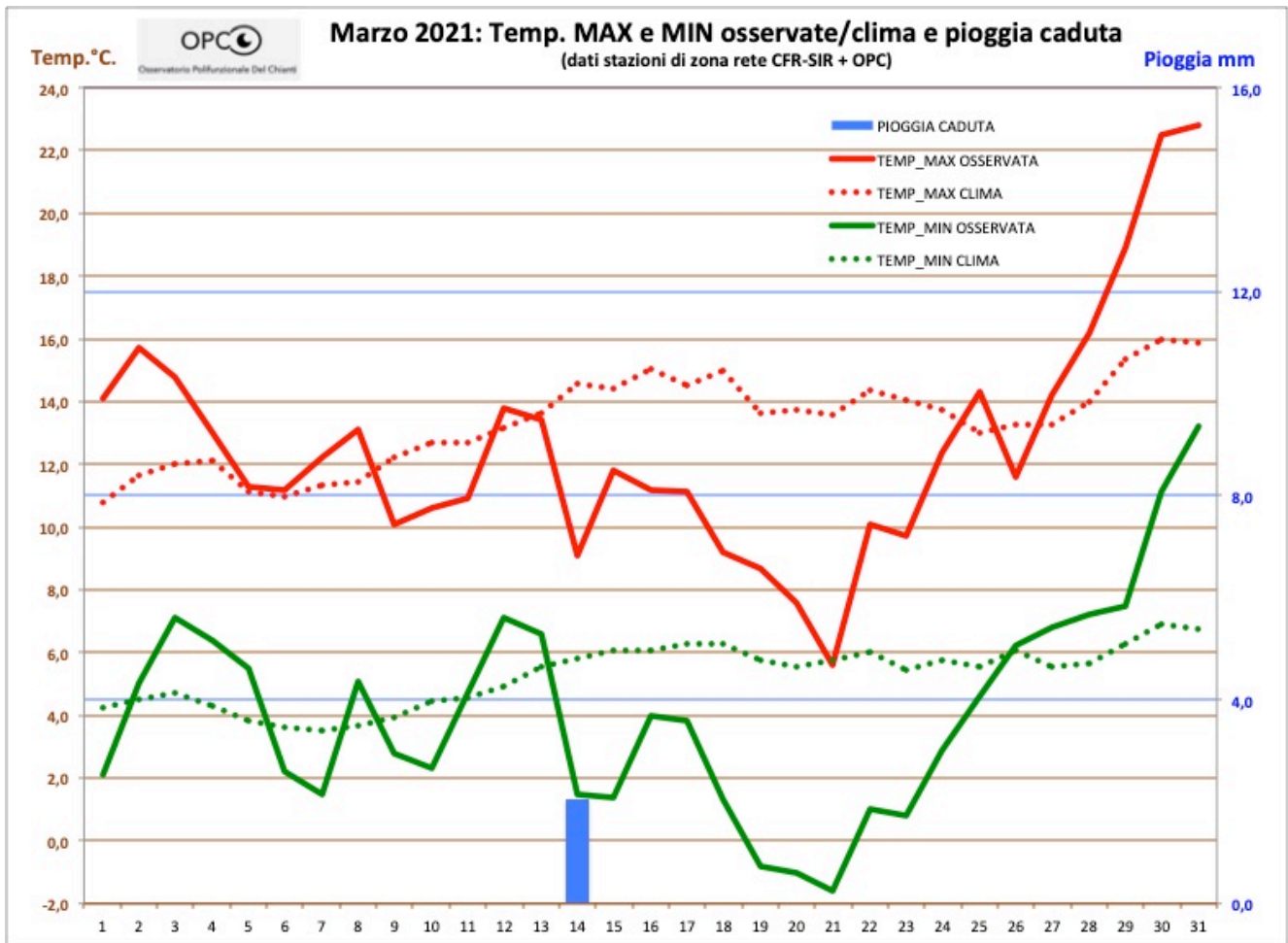
Andamento meteo climatico mese di MARZO 2021
